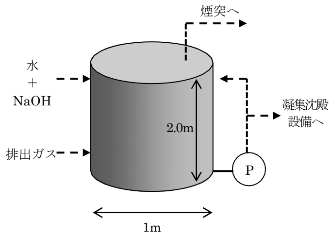
○図5 廃ガス洗浄施設の構造
