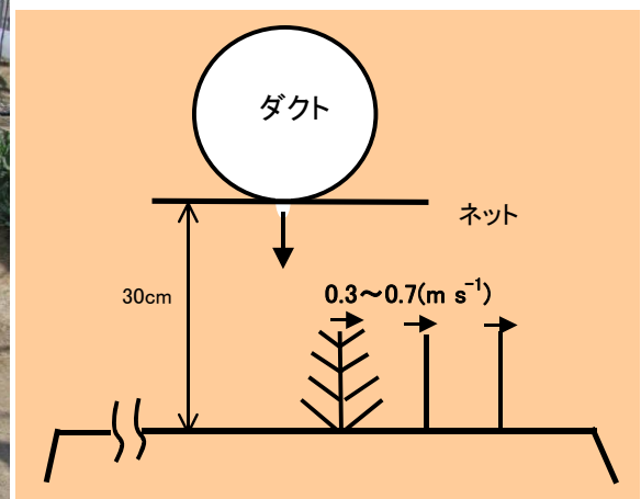
温風機(ダクト)を用いた送風方法
