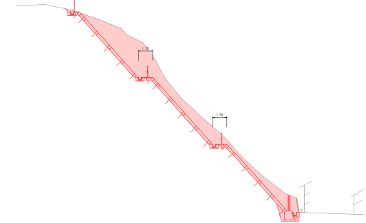
標準断面図
