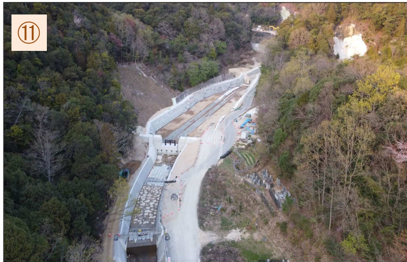
天地川（堆積工） 施工状況
