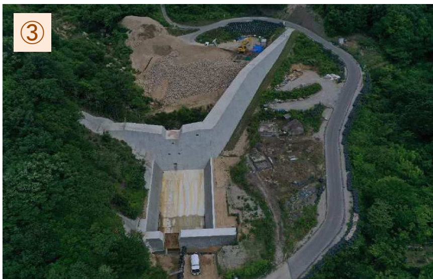
③ 天地川支川1 砂防堰堤（本体工）令和3年2月26日完成
