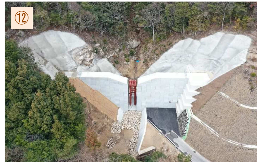
天地川支川3 令和5年2月28日完成
