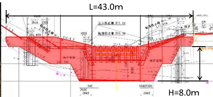
堰堤一般図
