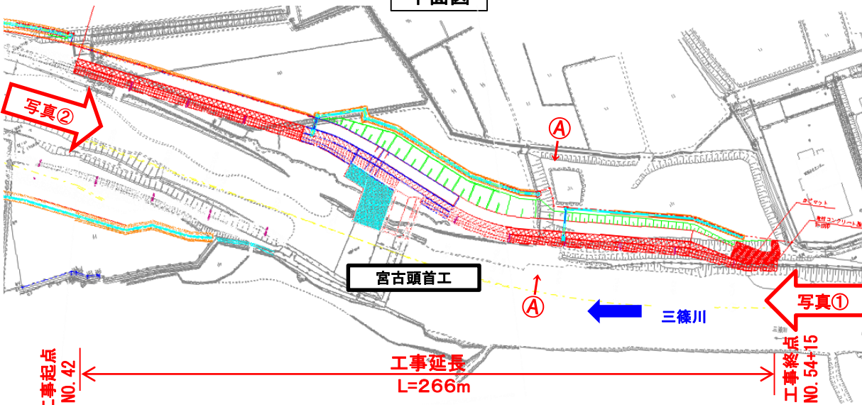
平面図
