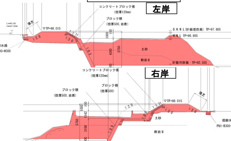
標準断面図 (A-A)
