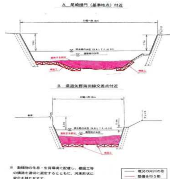
横断面
