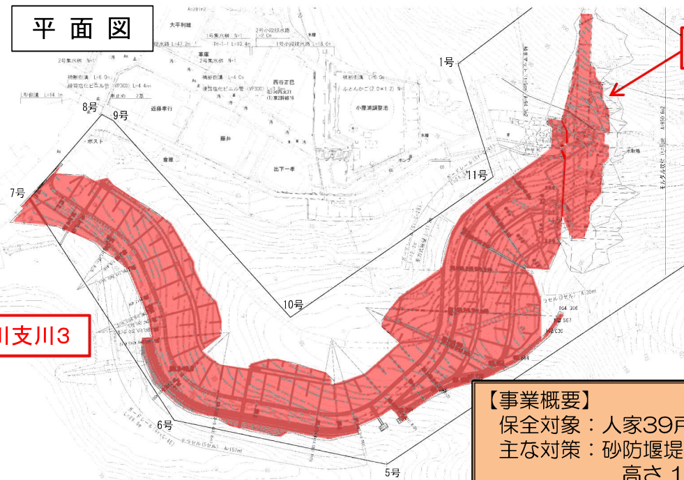
砂防堰堤
