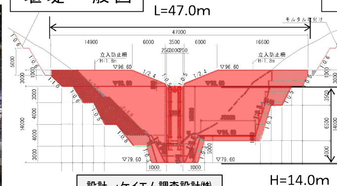
堰堤一般図
