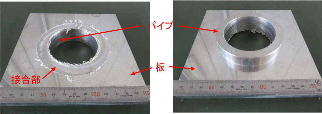
高速回転ホルダーで接合した板とパイプのL字継手外観写真
