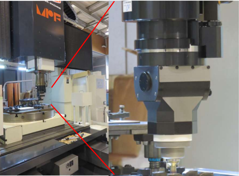
摩擦かくはん接合装置 高速回転ホルダー
