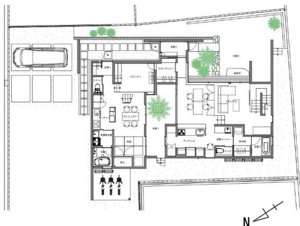
1階平面図
