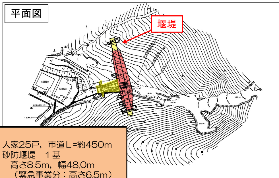
堰堤一般図
