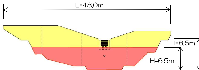
堰堤一般図
