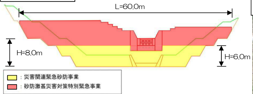
堰堤一般図
