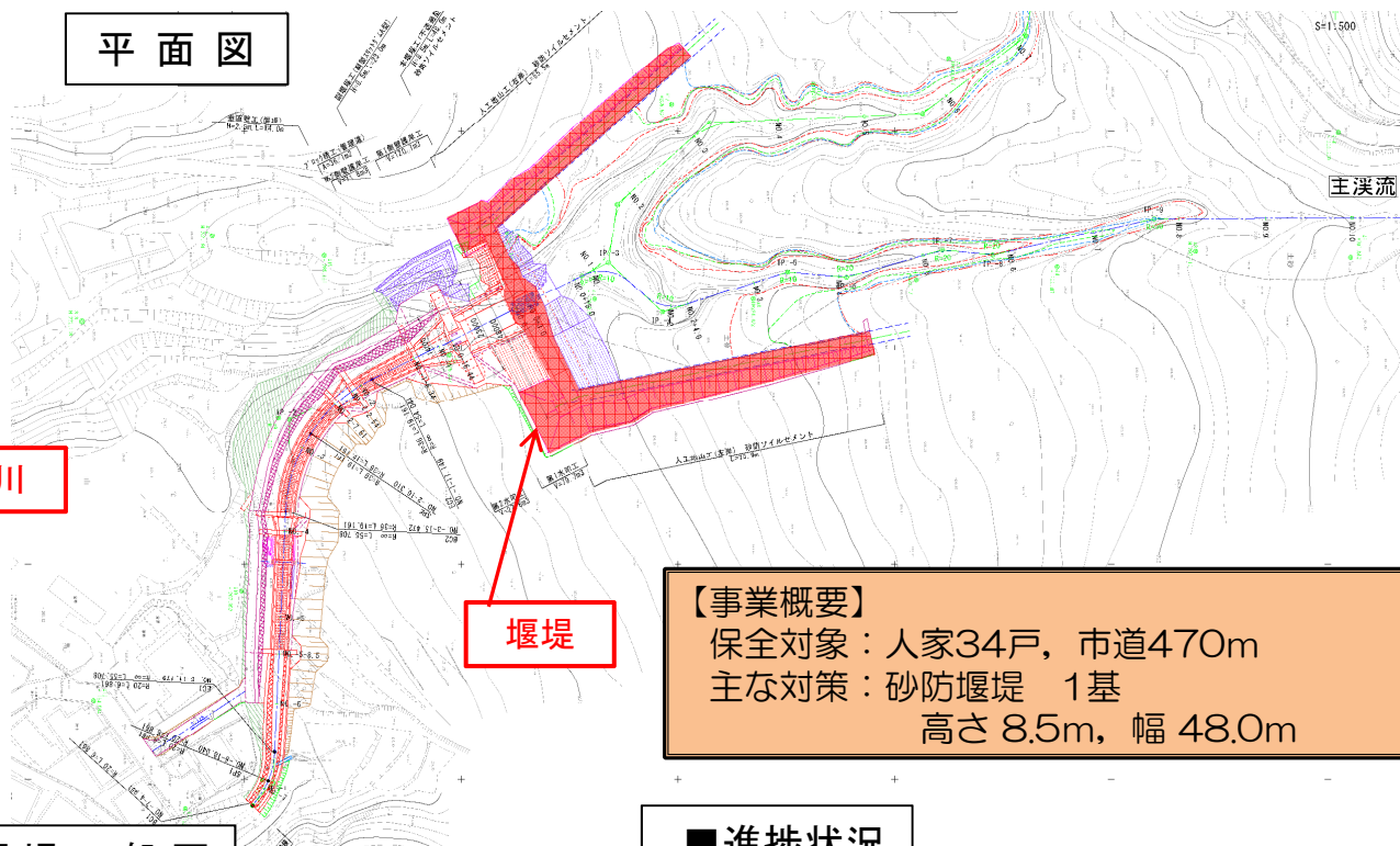
堰堤一般図
