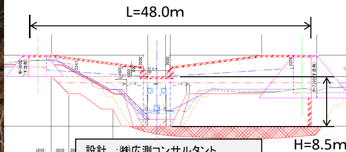
堰堤一般図
