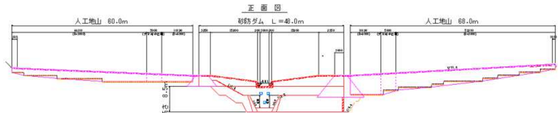
堰堤正面図
