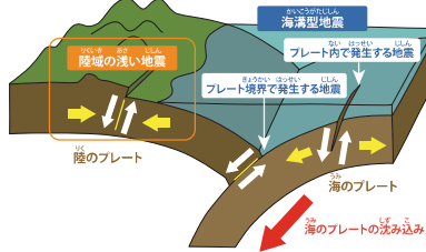
出典: 気象庁「地震の仕組み」に掲載されている「プレート境界」(注) http://www.jma.go.jp/jma/naohoku/naohoku/naohoku.html
