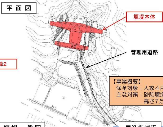
堰堤一般図
