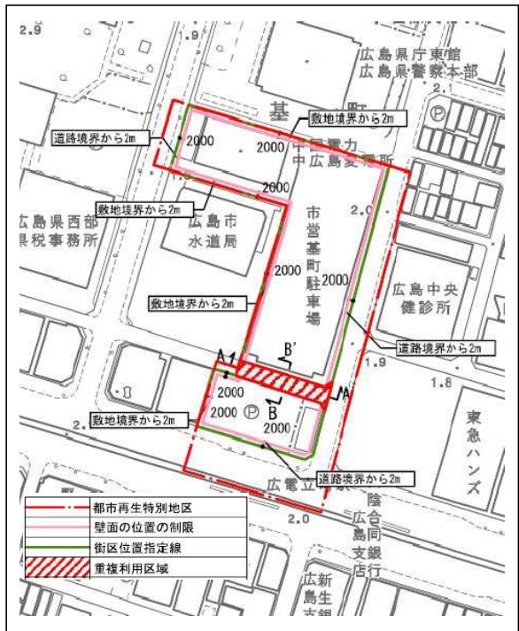
計画図
