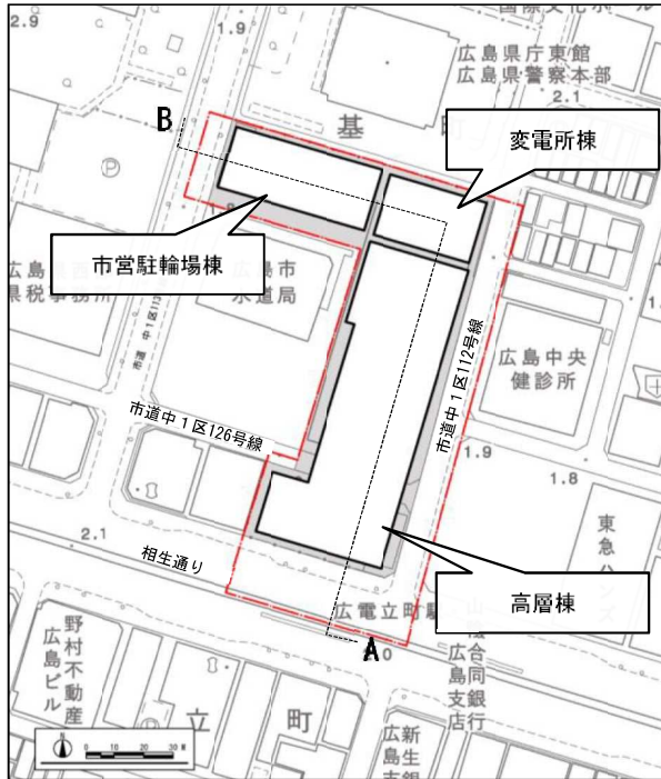
建物配置図
