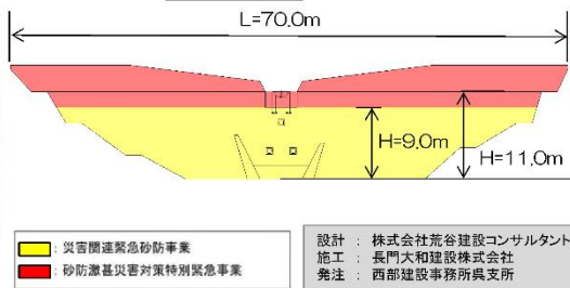
堰堤一般図
