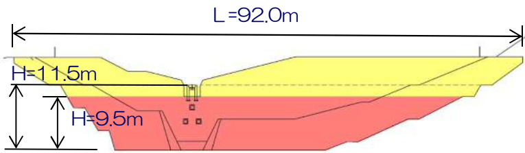
堰堤一般図
