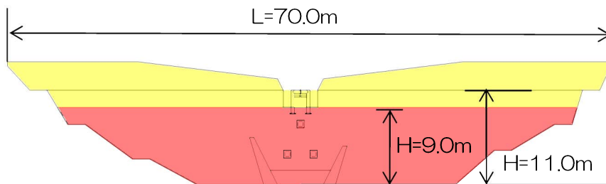
堰堤一般図
