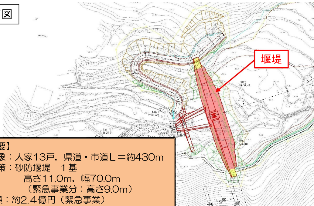
堰堤一般図
