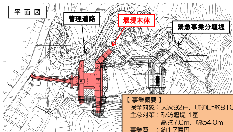
堰堤一般図
