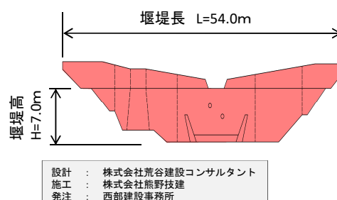
堰堤一般図
