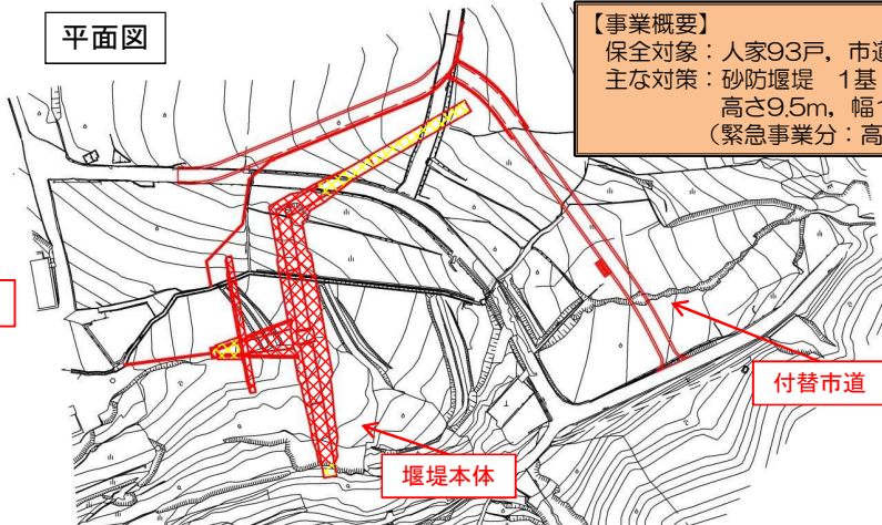
堰堤一般図
