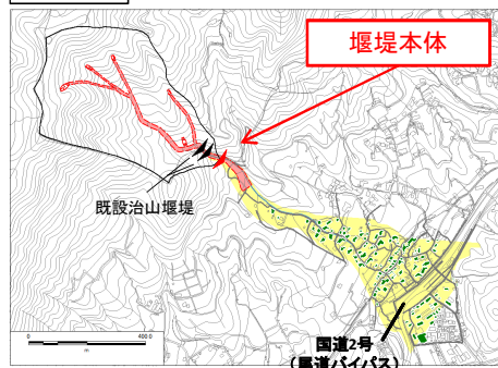
堰堤一般図
