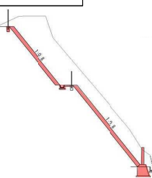
標準断面図
