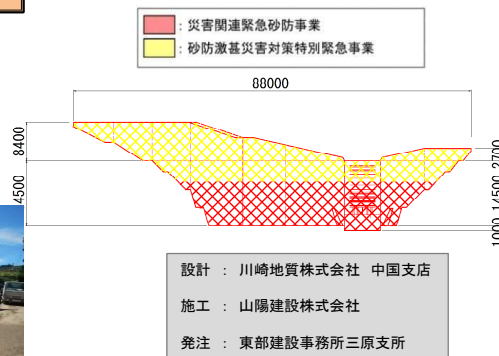
堰堤一般図
