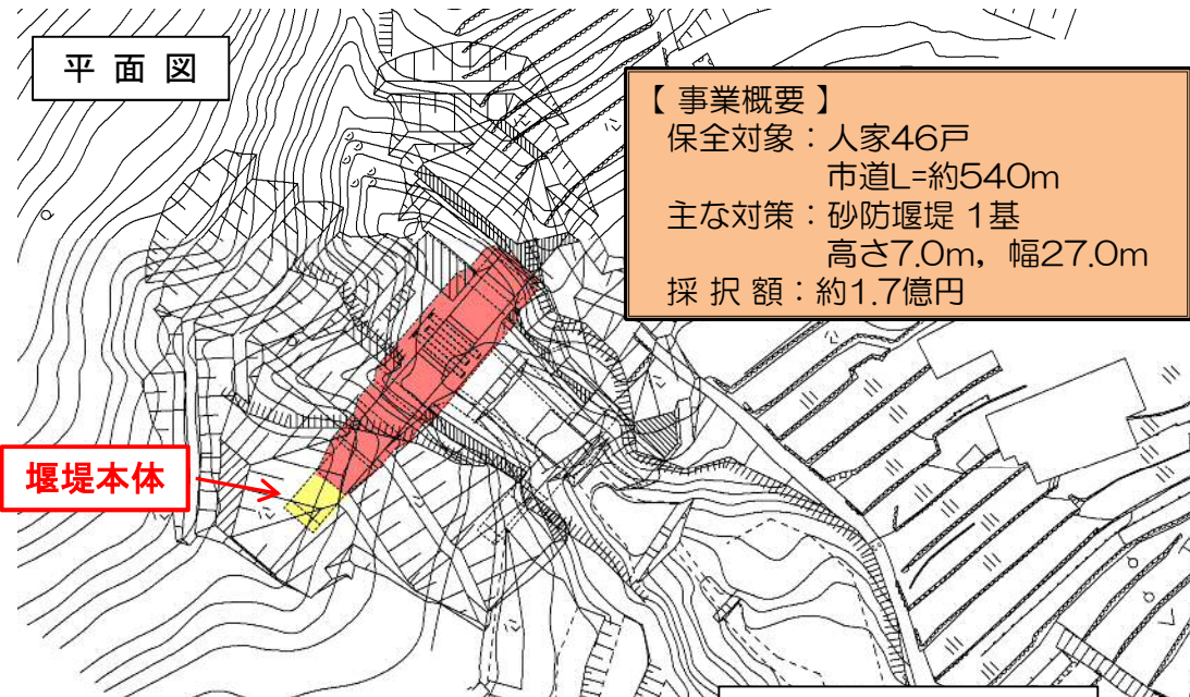
堰堤一般図
