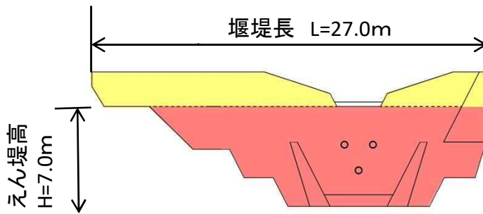
堰堤一般図
