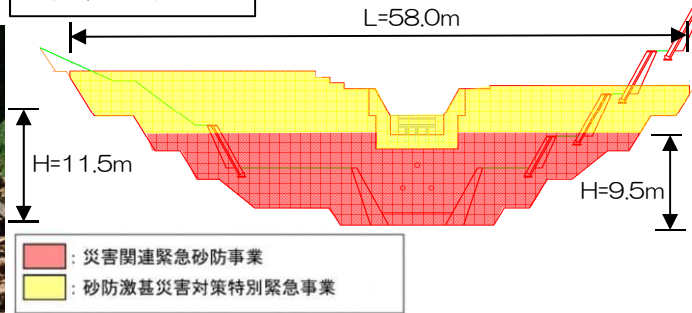
堰堤一般図
