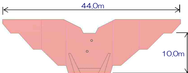
堰堤一般図
