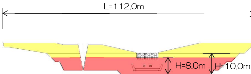
堰堤一般図
