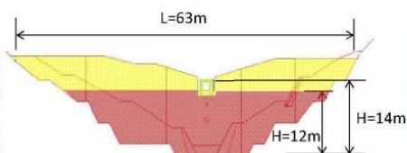
堰堤一般図
