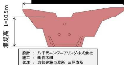
堰堤一般図
