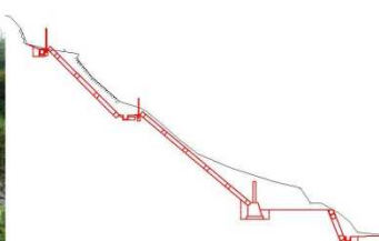
標準断面図
