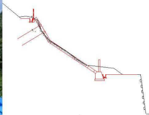
標準断面図
