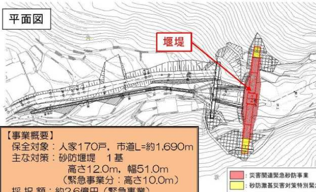
堰堤一般図
