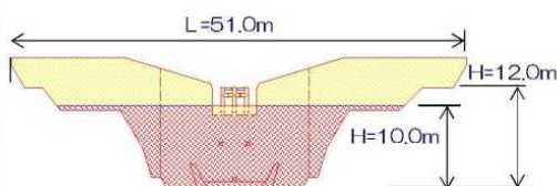
堰堤一般図
