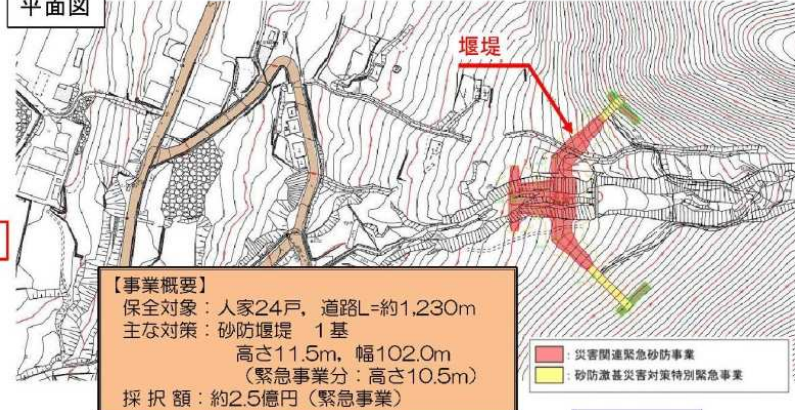
平面図
