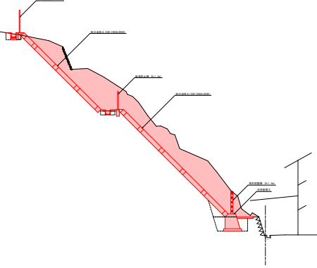
標準断面図
