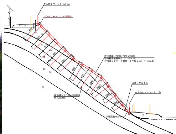
標準断面図
