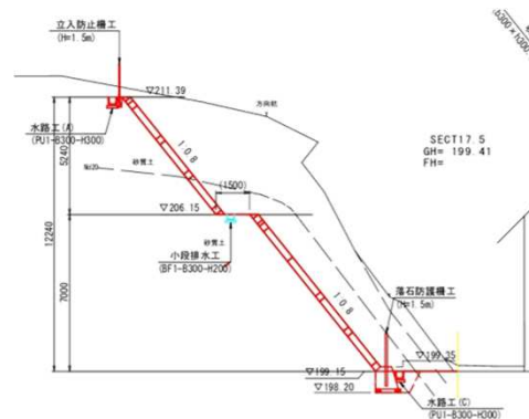
標準断面図
