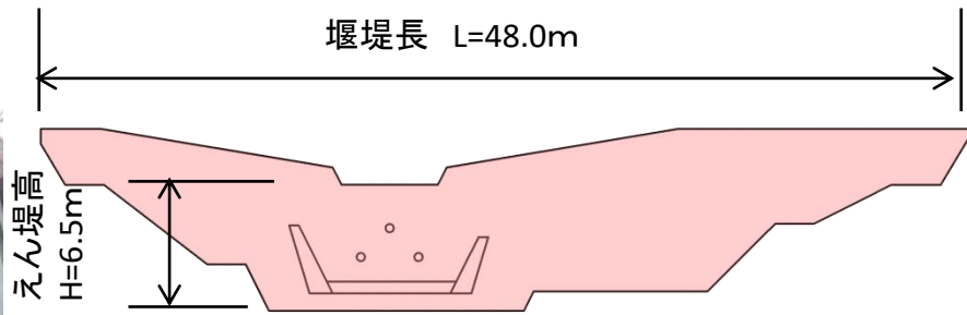
堰堤一般図
