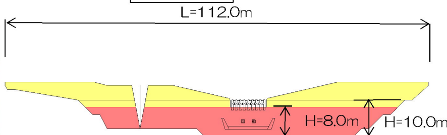
堰堤一般図
