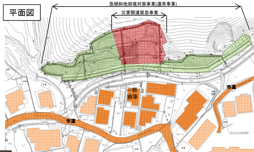
斜面崩壊・被災状況（H30年7月）
