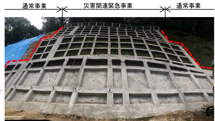
工事完了（令和2年8月11日）
