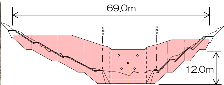
堰堤一般図
