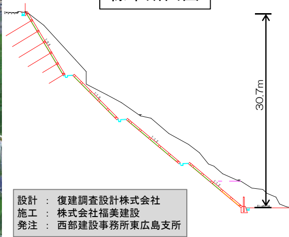
標準断面図
