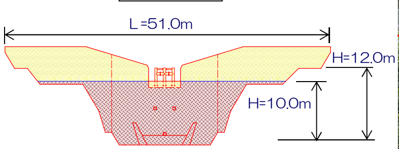
堰堤一般図
