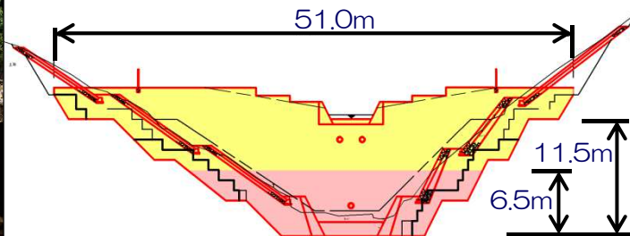
堰堤一般図
