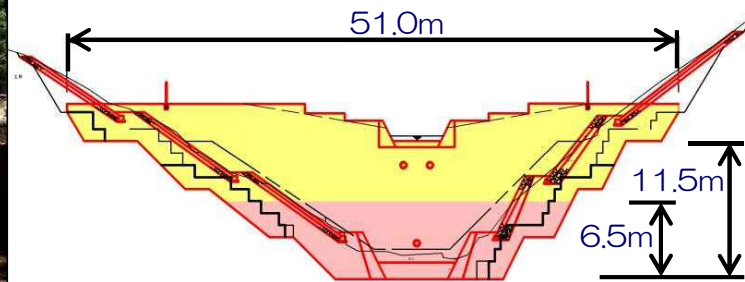
堰堤一般図
