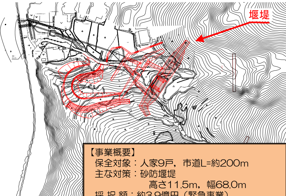
堰堤一般図
