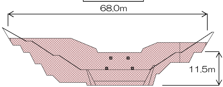
堰堤一般図
