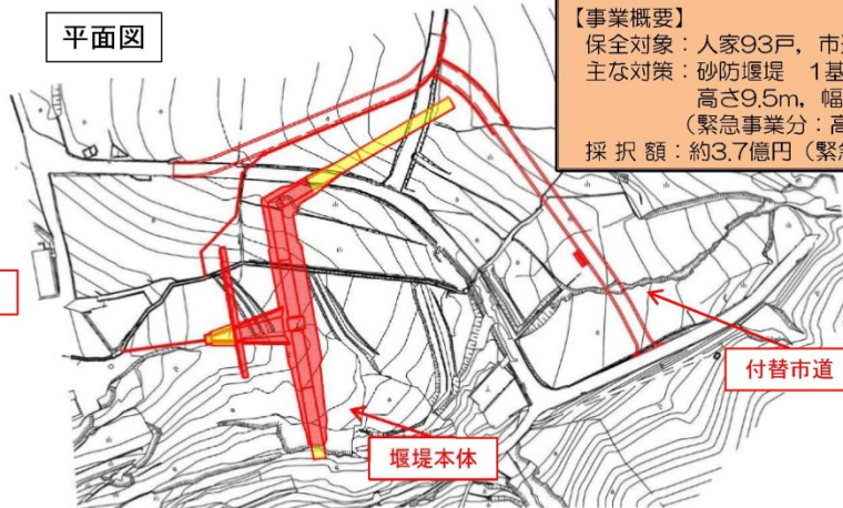
堰堤一般図
