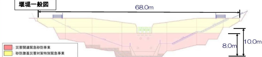
堰堤一般図
