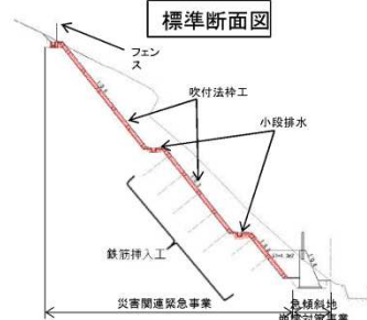
標準断面図
