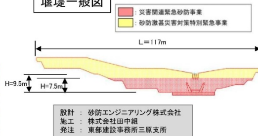
堰堤一般図
