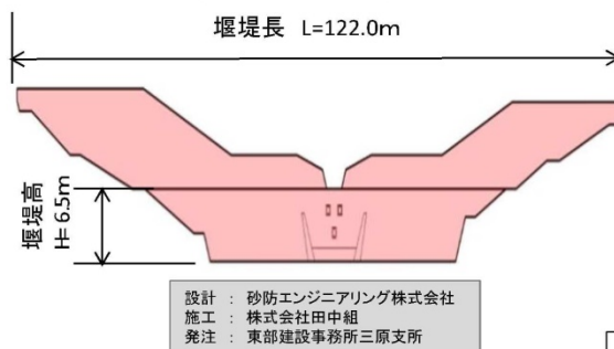
堰堤一般図
