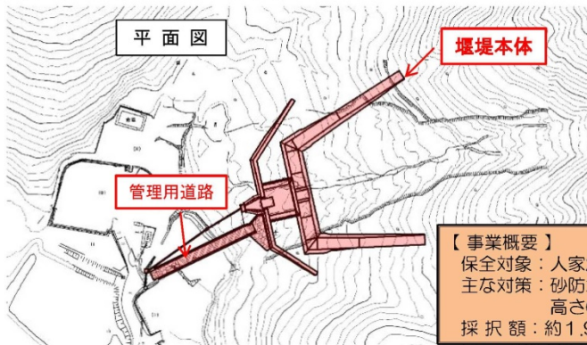
堰堤一般図
