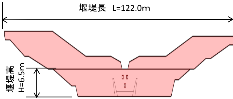
堰堤一般図
