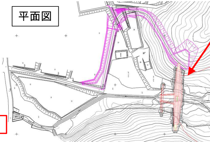
堰堤一般図
