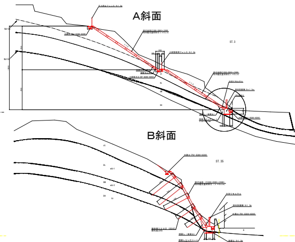
標準断面図
