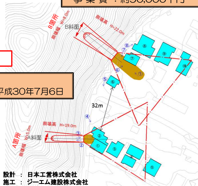
平面図
