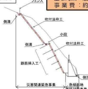
標準断面図
