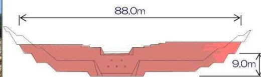
堰堤一般図
