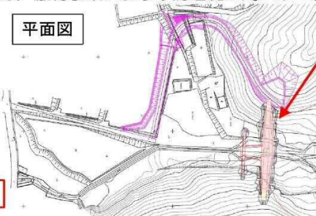
堰堤一般図
