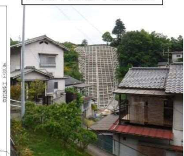
工事完了（令和2年6月30日）
