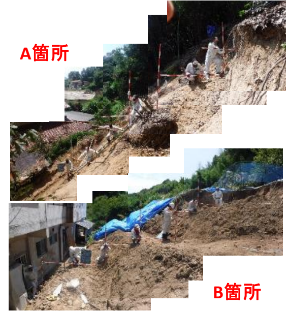
斜面崩壊・被災状況（H30年7月）
