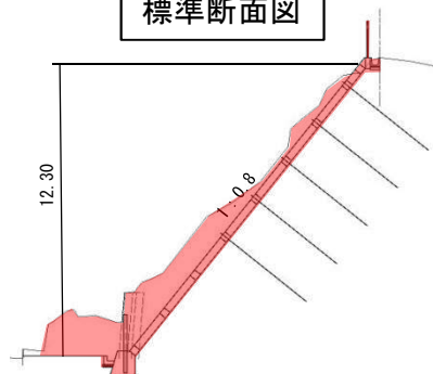
標準断面図
