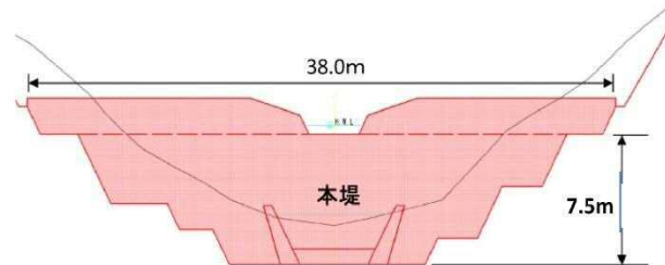
堰堤一般図
