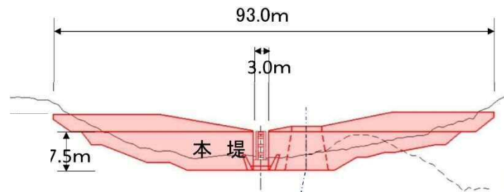
堰堤一般図
