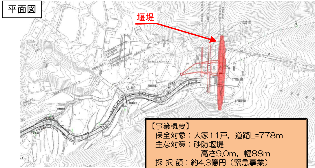
堰堤一般図
